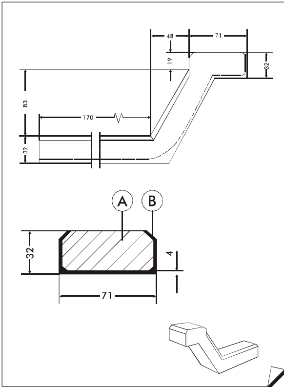
Gummi formstück 3 Way Watertight Joint 3 Yönlü Köşe Kauçuk
